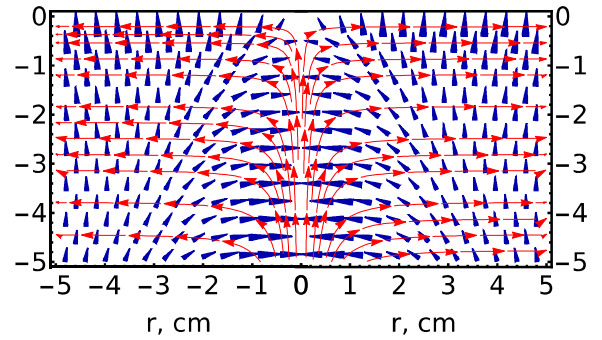
Рис. 7. Вектор Пойтинга \mathbf{S}_p в начальный момент времени, определенный с помощью закона Ома с проводимостью \sigma (22). Структура полоидального тока \mathbf{j}_p показана красными стрелками.
