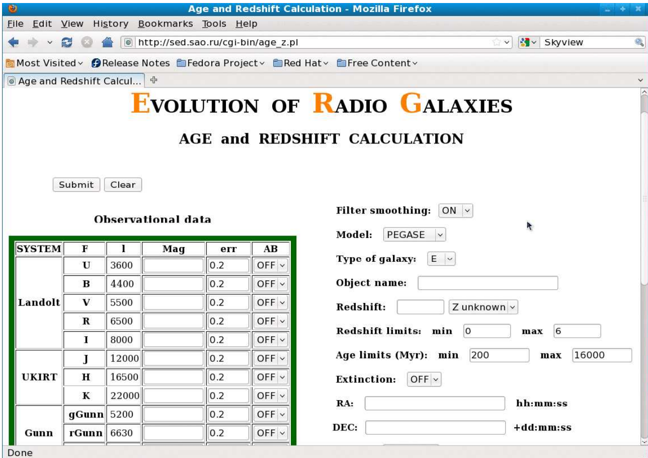
Рис. 7: Web-страница SED с формой ввода фотометрических измерений для оценки возраста.
