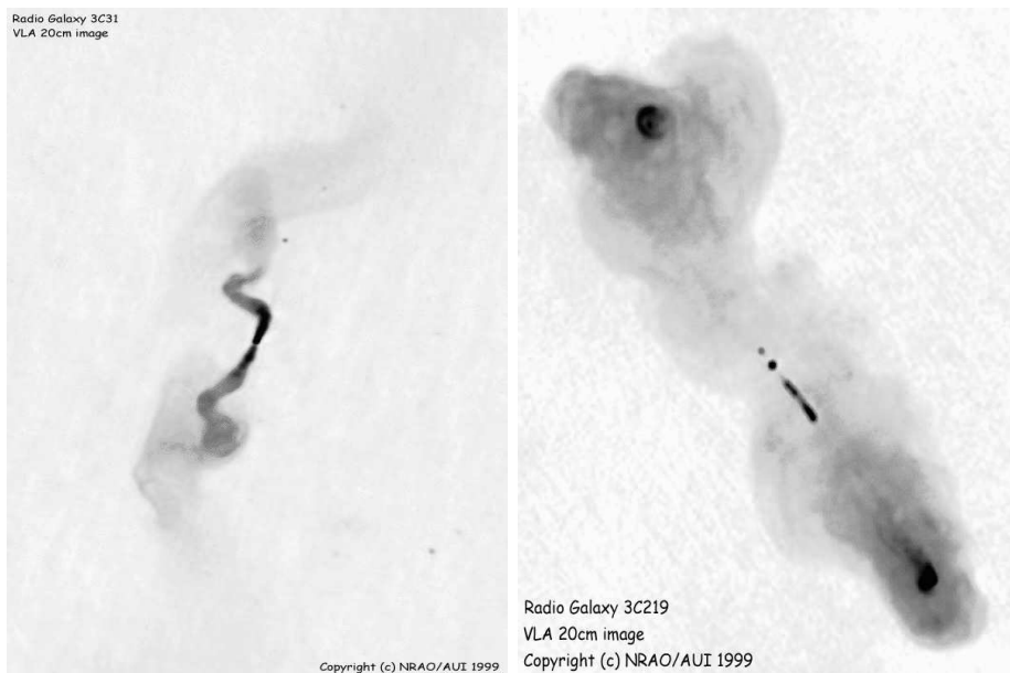
Рис. 1: Слева: изображение радиогалактики 3C 31, относящейся к классу FR I. Справа: изображение радиогалактики 3C 219, относящейся к классу FR II. Рисунки воспроизведены с сайта http://www.cv.nrao.edu/~abridle/images.htm .
